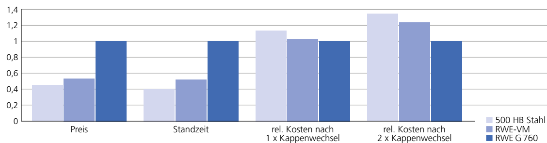
Vergleich unterschiedlicher Materialien beim Einsatz in Schwertwäschen
